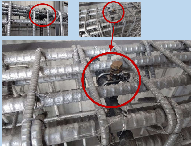
梁受け架台使用例
